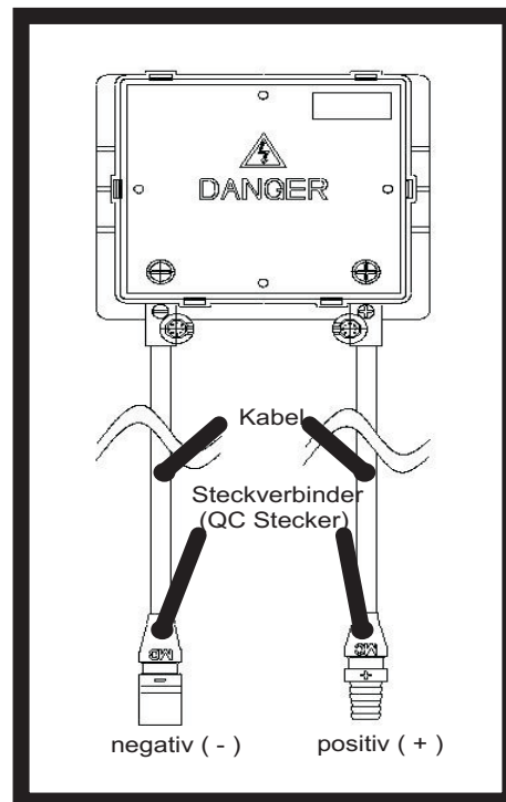
Abb 3: Konfiguration der Anschlussdose
